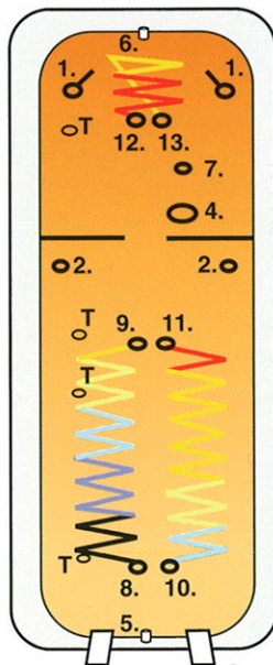
Akvair Solar 500, 750, 1000
