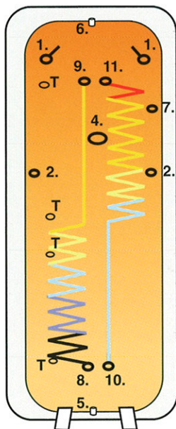
Akvair Solar 300
